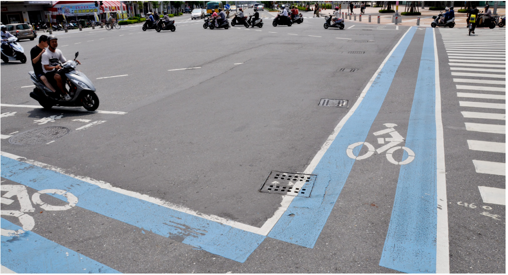
Foto 22. Demarcación intersección cruce de ciclistas. Arriba, Kaohsiung, China. Fuente: Carlos Felipe Pardo. Abajo, Copenhague. Fuente: Patricia Calderón.
