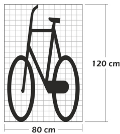
Figura 32. Pictograma bicicleta en ciclovía, ciclocarril o cicloacera y localización con respecto a la esquina.. Fuente: Ministerio de Transporte de Colombia, 2016
