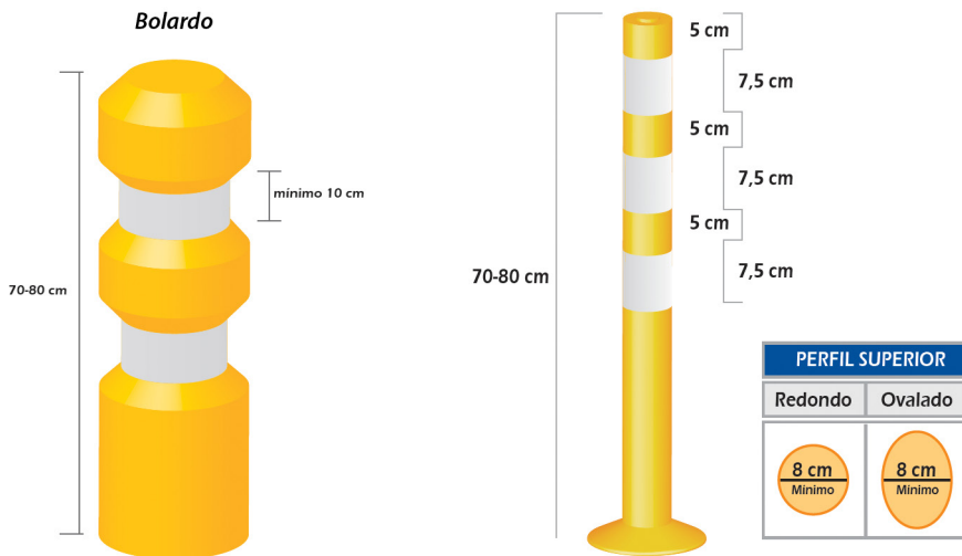
Figura 41. Bolardos. Fuente: Ministerio de Transporte de Colombia, 2016
