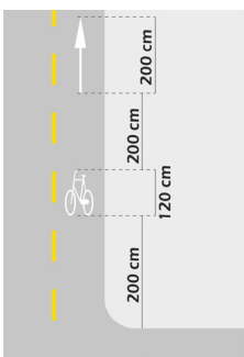
Figura 32. Pictograma bicicleta en ciclovía, ciclocarril o cicloacera y localización con respecto a la esquina.. Fuente: Ministerio de Transporte de Colombia, 2016
