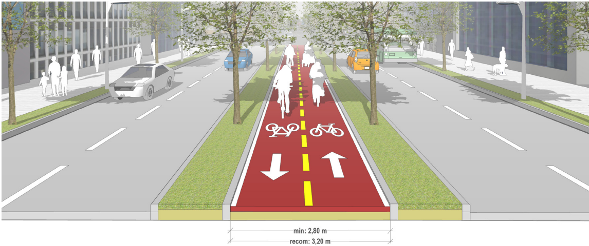
Figura 13. Ejemplo esquemático de ciclovia (bidireccional) en separador central
