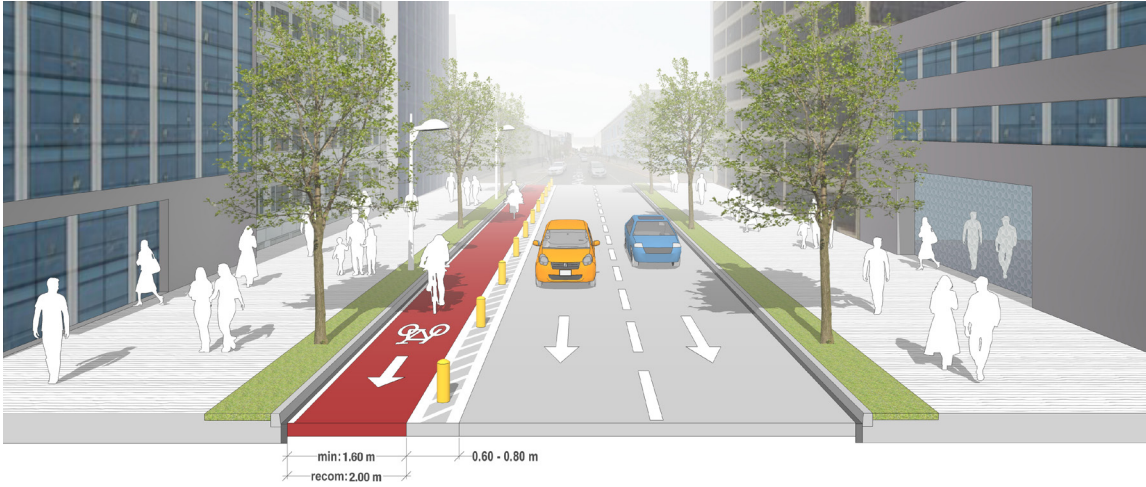
Figura 12. Ejemplo esquemático de ciclovia unidireccional
